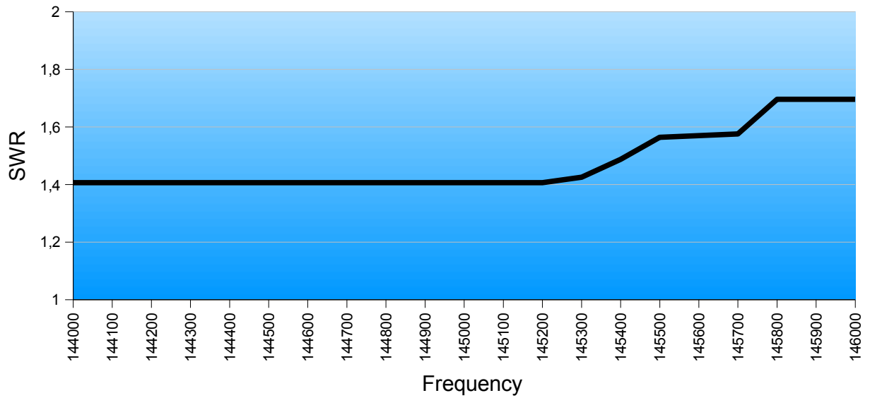
2 meter SWR Chart ON3JT
